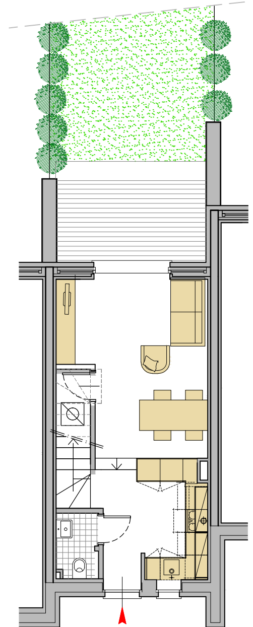
PIANO TERRA GROUND FLOOR первый этаж
